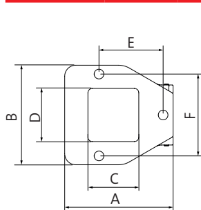
Wymiary / Otwór montażowy FWS-B 11 do 21
