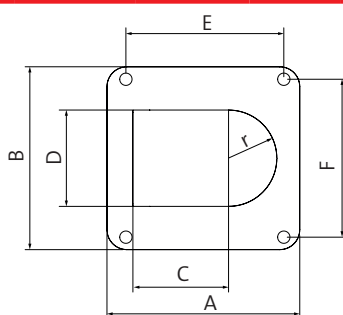
Wymiary / Otwór montażowy FWS-B 29 do 48
