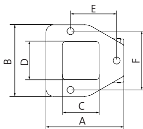
Wymiary / Otwór montażowy FWS-A 16 do 25
